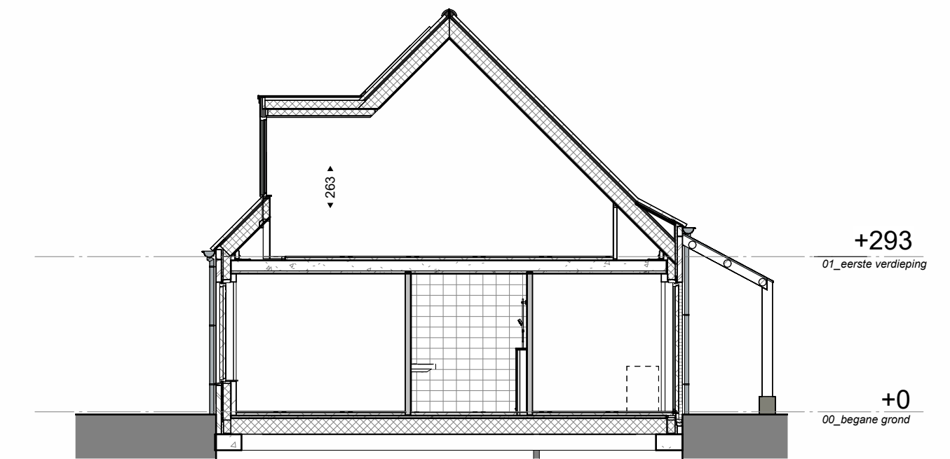
dwarsdoorsnede F2
